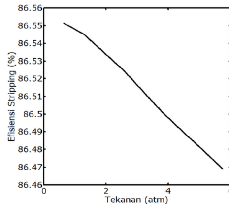
Gambar 4. Pengaruh tekanan stripper terhadap % efisiensi kolom stripping
